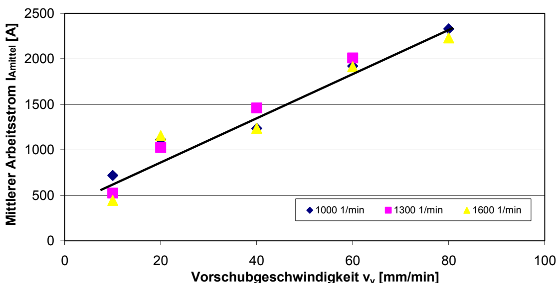
Bild 5.7: Mittelwert des Arbeitsstroms I_{Amittel} in Abhängigkeit von der Vorschubgeschwindigkeit v_v bei unterschiedlichen Drehzahlen ( H = 80 mm, v_v 10 - 80 mm/min, Werkstoff 1.4301)
