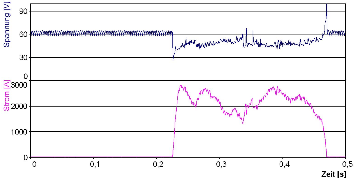
Bild 5.17: Typischer CAMC-Prozessverlauf, mit unregelter Stromquelle ( H = 80 mm, v_v = 40 mm/min, Werkstoff 1.4301, Stromquelle CG 2000)
