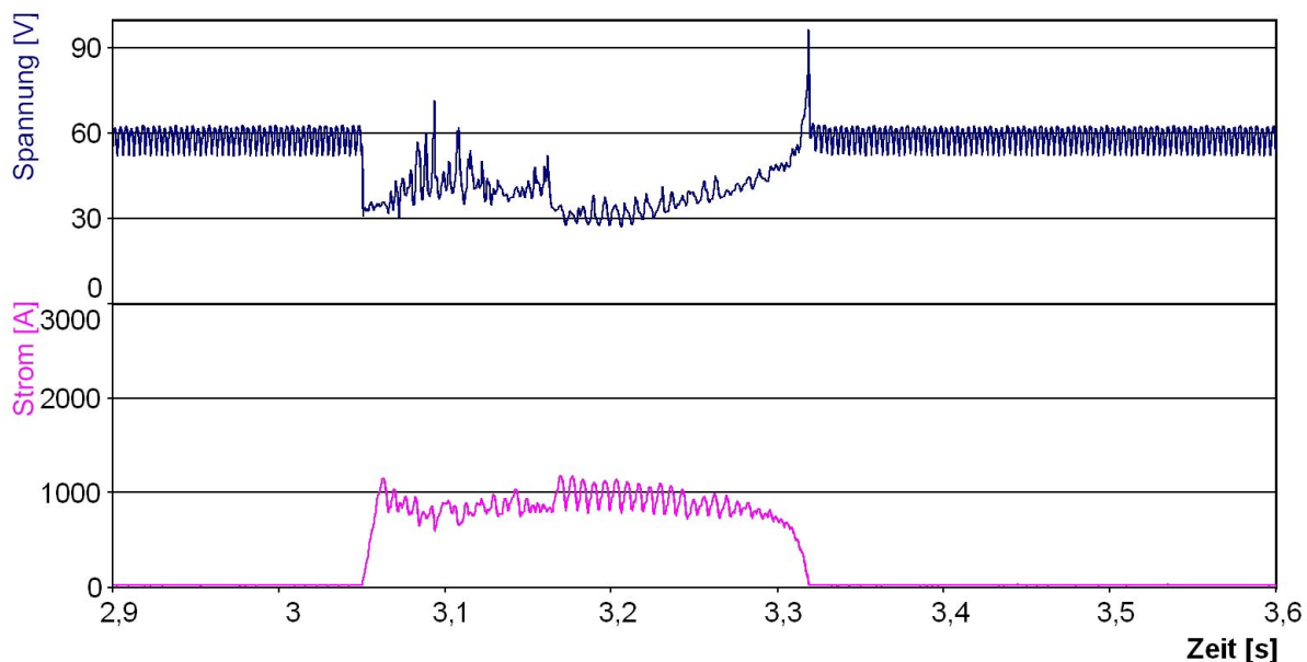
Bild 5.18: Typischer CAMC-Prozessverlauf, mit geregelter Stromquelle ( H = 80 mm, v_v = 5 mm/min, Werkstoff 1.4301, Stromquelle GTH 802)
