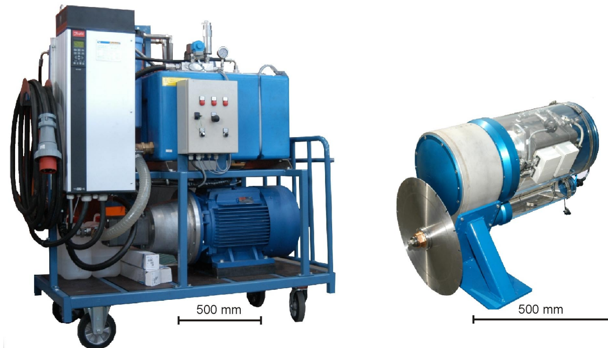
Bild 4.2: Wasserhydraulikaggregat (links), CAMG-Werkzeug (rechts)
