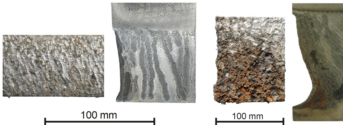
Bild 5.23: CAMC-Schnittfugenflächen und –Elektroden bei starker Spülströmung (links) und bei schwacher Spülströmung (rechts)
