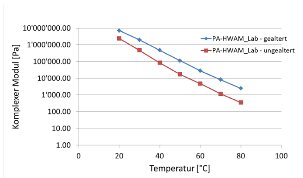
Abb. 52 Komplexer Modul (DSR) der Labormischung PA-HWAM gealtert/ungealtert bei einer Frequenz von 1.6 Hz und unterschiedlichen Temperaturen
