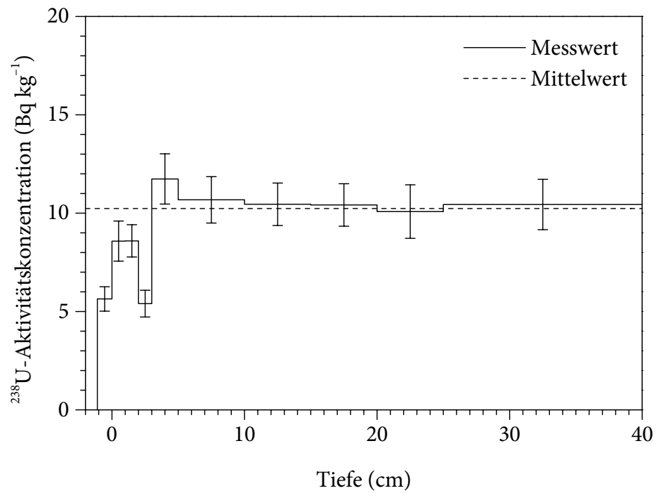
Abb. 94: ^{238}\text{U} -Aktivitätskonzentration in Abhängigkeit von der Tiefe im Bodenprofil »Woronowo«
