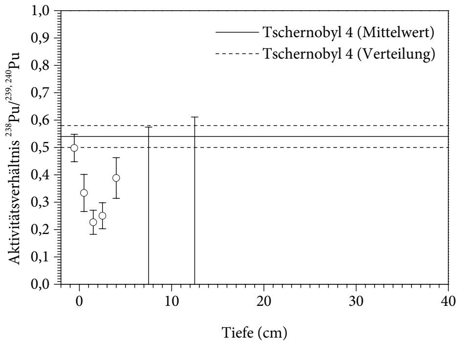
Abb. 99: 238 Pu/ 239,240 Pu-Aktivitätsverhältnis in Abhängigkeit von der Tiefe im Bodenprofil »Woronowo«. Die Unsicherheiten sind erweiterte Standardunsicherheiten ( k = 2 ).
