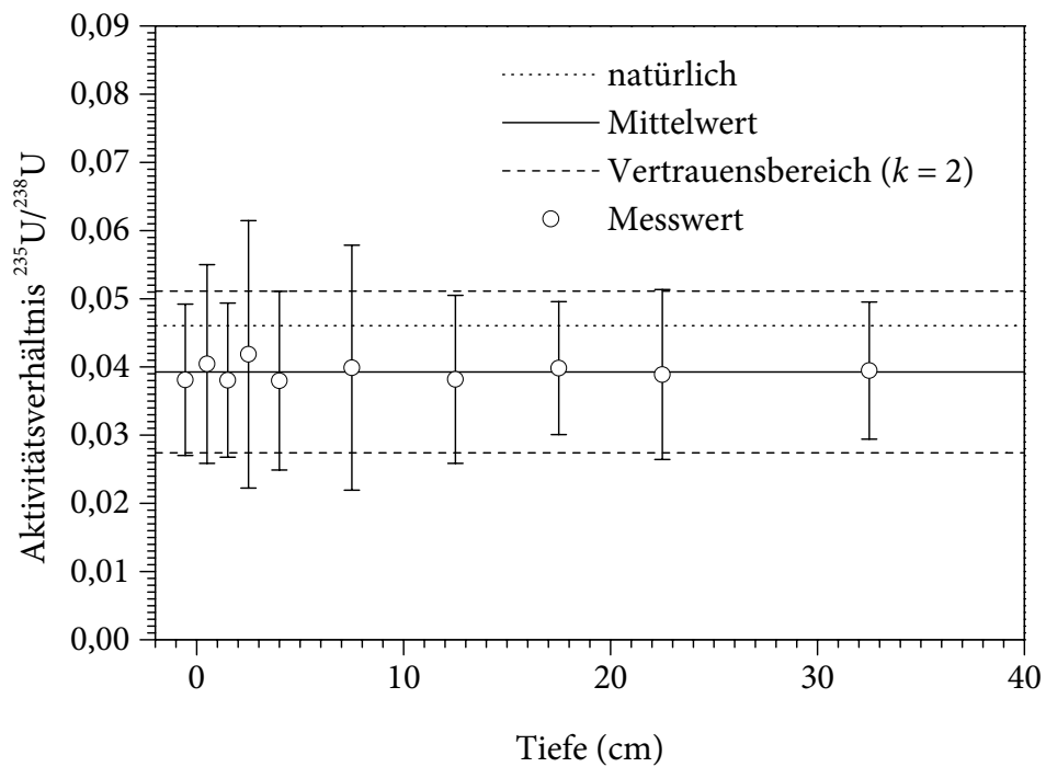
Abb. 95: ^{235}\text{U}/^{238}\text{U} -Aktivitätsverhältnis in Abhängigkeit von der Tiefe im Bodenprofil »Woronowo«. Die Unsicherheiten sind erweiterte Standardunsicherheiten ( k = 2 ).
