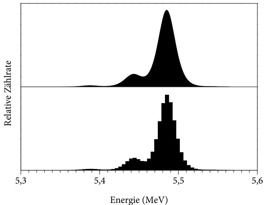
Abb. 49: Theoretische Gestalt des \alpha -Spektrums von ^{241}\text{Am} ( E_{\alpha} = 5\,485,6 keV; P_{\alpha} = 85,2 %) vor (oben) und nach der Digitalisierung mithilfe eines Analog-Digital-Wandlers (unten), bei einer elektronischen Auflösung von 17 keV und einer Kanalbreite von 4,56 keV.
