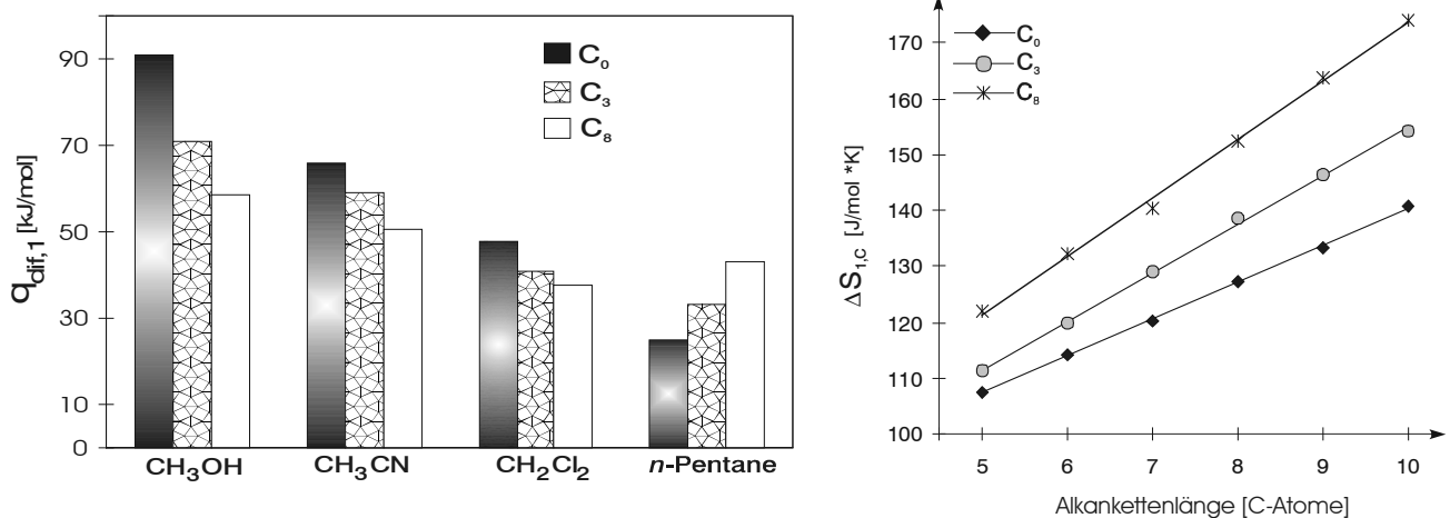
Abb. 40: Differentielle Adsorptionswärme (links) und Differentielle Adsorptionsenthalpie (rechts) von molekularen Sonden auf polarer Kieselsäure (C 0 ) und silanisierter Kieselsäure (C 3 , C 8 )
