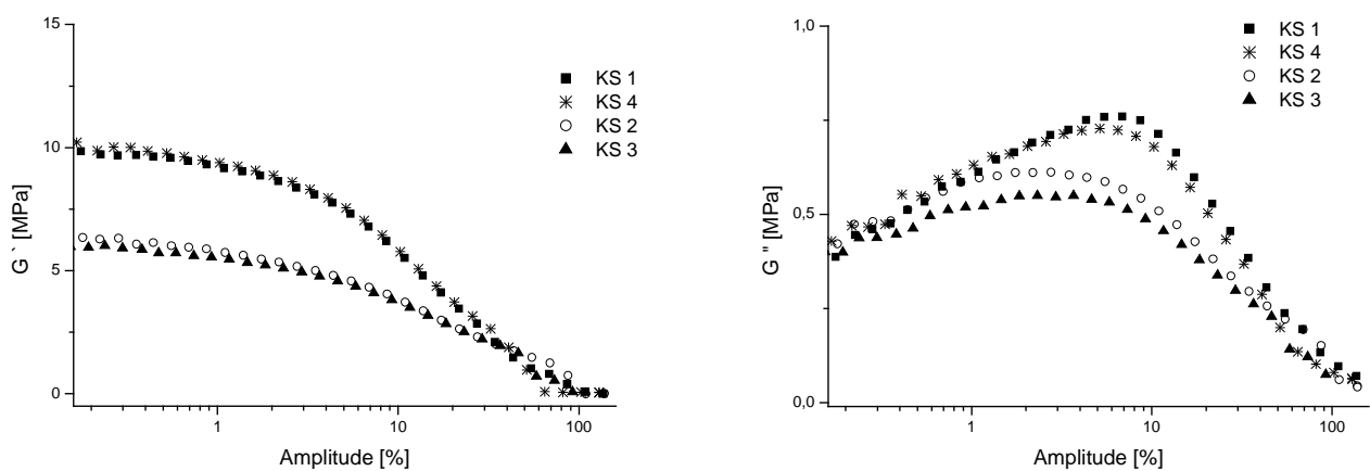
Abb. 48: Amplitudenabhängigkeit der Moduli („Payne-Effekt“)
