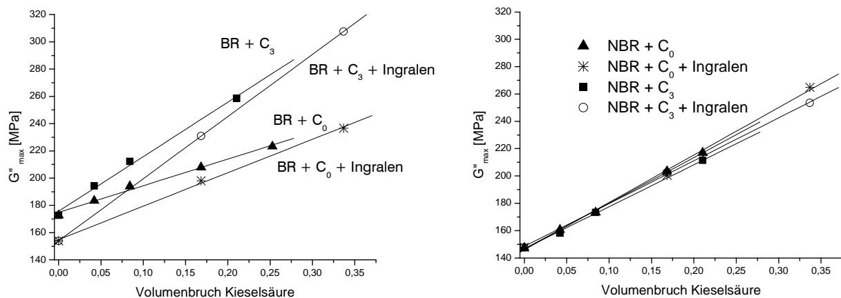
Abb. 65: Einfluss des Weichmacheröls Ingralen auf den maximalen Verlustmodul
