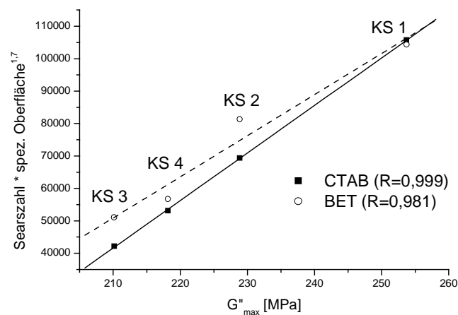
Abb. 47: Abhängigkeit der maximalen Dämpfungsamplitude von der spez. Oberfläche und der Oberflächenpolarität (SEARS-Zahl)
