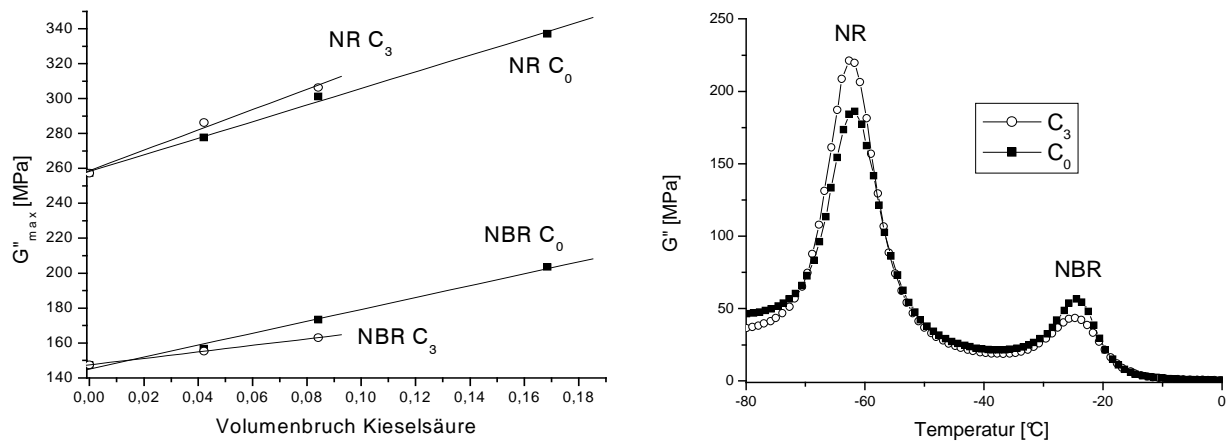
Abb. 68: Änderung des Verlustmoduls beim Einsatz silanisierter Kieselsäure
