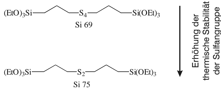
Abb. 27: Thermische Stabilität der Sulfangruppen
