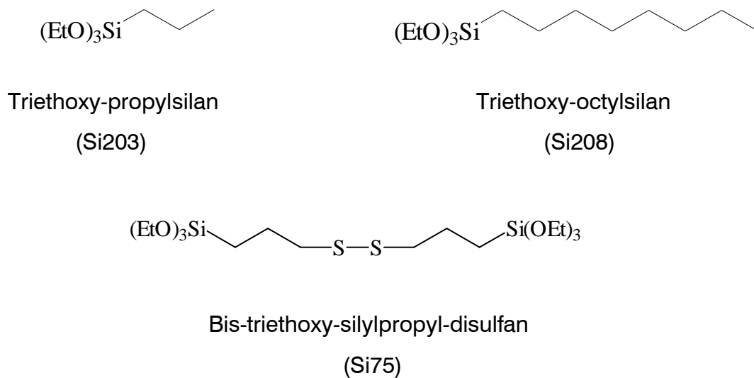
Abb. 30: Verwendete Silane
