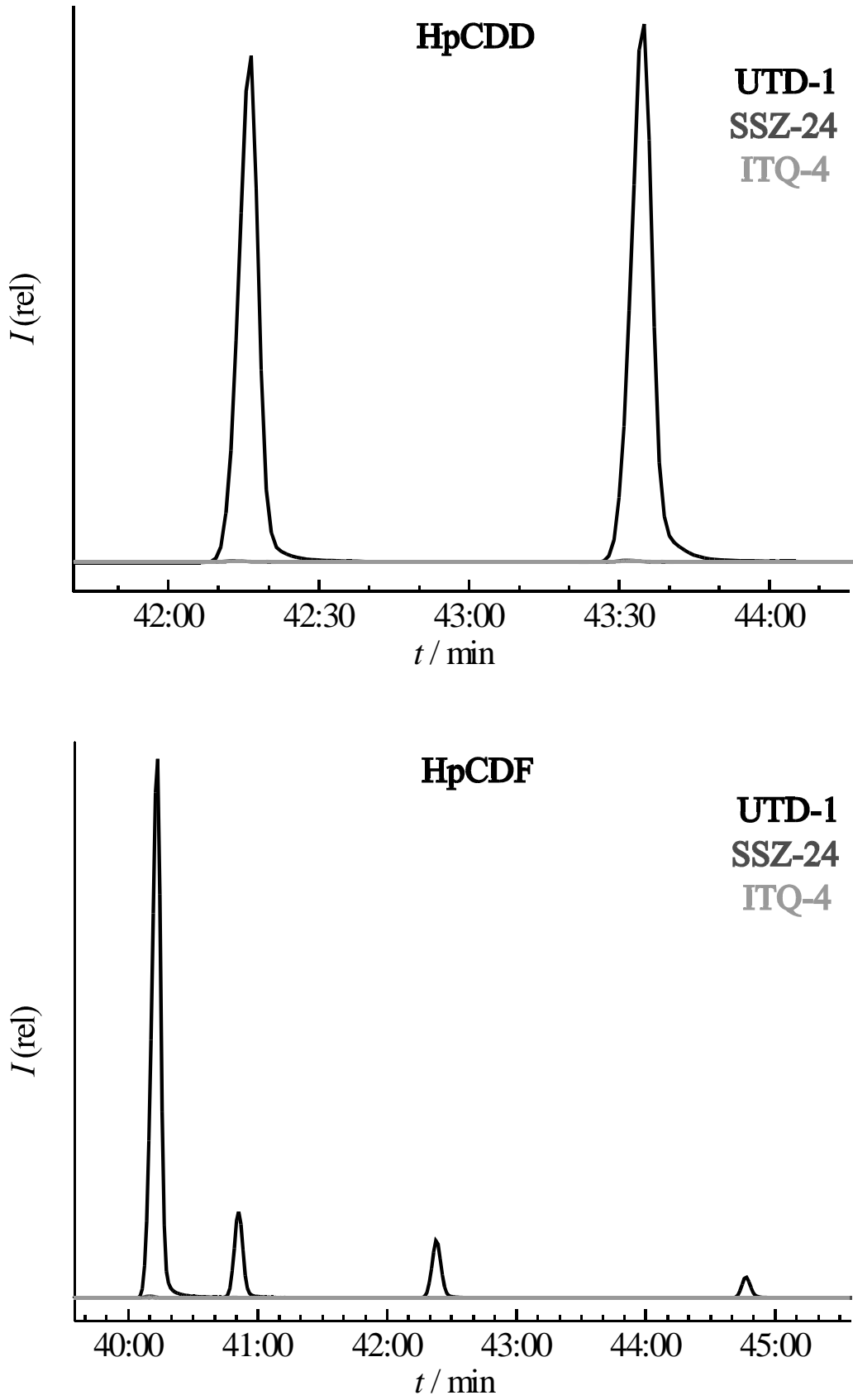
Abbildung 4.76. Versuch 9 Teil 7, HpCDD/F: Gaschromatogramme der extrahierten Proben.
