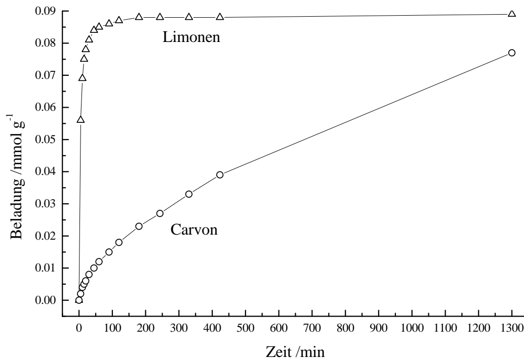
Abbildung 4.82. Adsorptionskinetik von Limonen und Carvon an ZSM-5 (aus LATZA [9] ).
