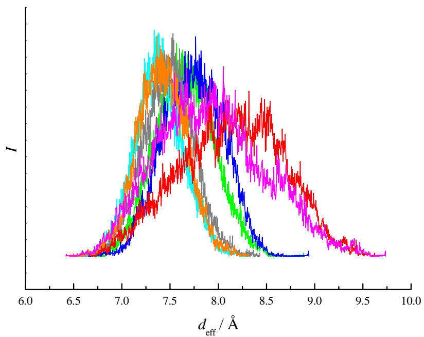
Abbildung 4.46. Verteilung einzelner effektiver Porendurchmesser aus der Simulation der Gerüstdynamik von CIT-5 bei 450 K.
