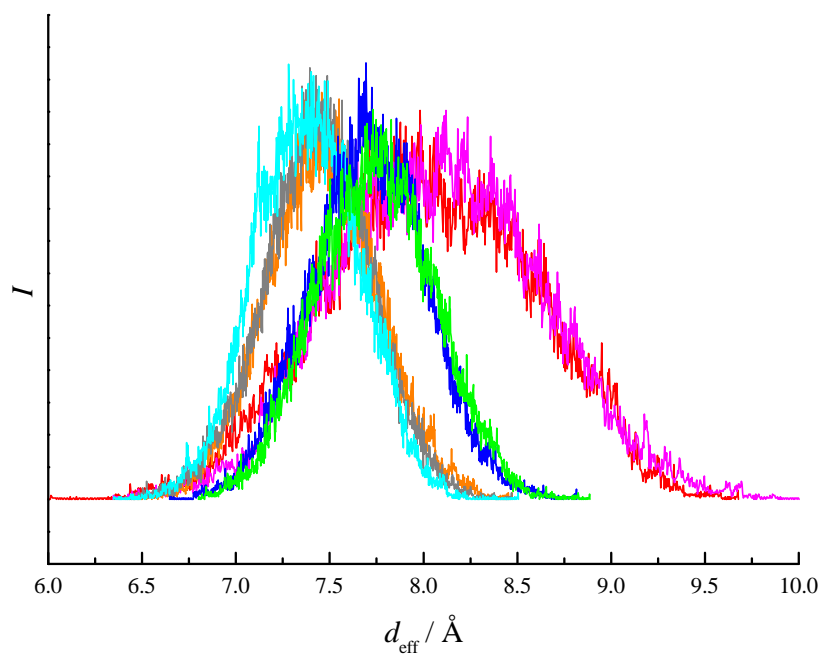
Abbildung 4.47. Verteilung einzelner effektiver Porendurchmesser aus der Simulation der Gerüstdynamik von CIT-5 bei 573 K.
