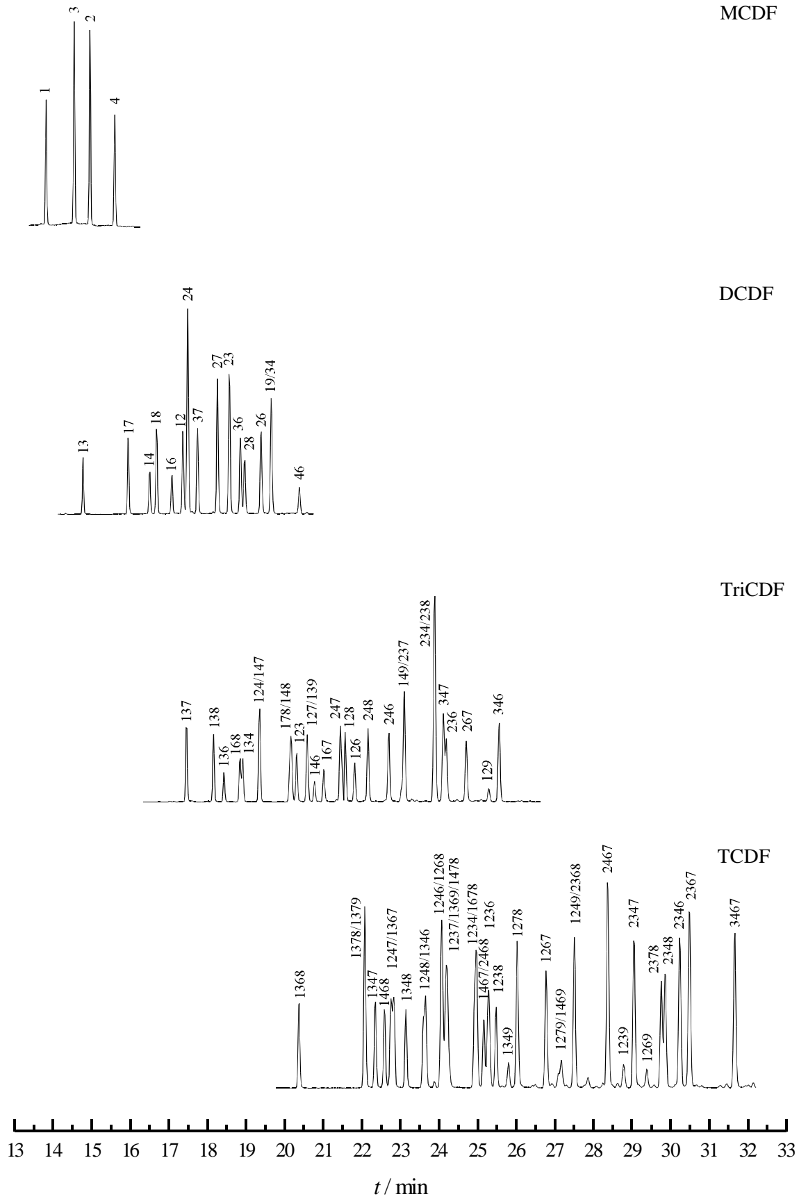
Abbildung 3.8. Zuordnung der mono- bis tetrachlorierten Dibenzofurane.
