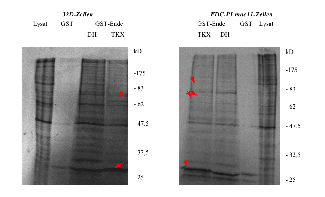
Abb. 3-25. Autoradiogramm von GST-pull-down-Experimenten mit Zellysaten metabolisch, ^{35}\text{S} -markierter 32D.C10- und FDC-P1 mac11-Zellen. Auf ein 11 %-iges SDS-Polyacrylamid-Gel wurden Proteinmarker, die jeweiligen Zellysate, sowie die jeweiligen Ansätze der GST-pull-down-Experimente aufgetragen. Die roten Pfeile markieren die Positionen der spezifischen Bindproteine.
