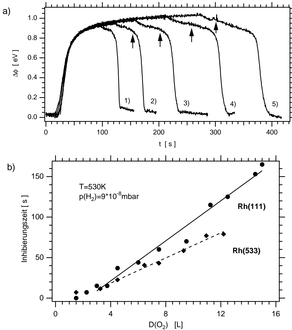
Abbildung 3.9: a) Austrittsarbeitsänderung bei der Dosierung von \text{Rh}(533) mit \text{O}_2 . Der Pfeil kennzeichnet den Zeitpunkt an dem p(\text{H}_2) = 9 \cdot 10^{-8} mbar eingestellt wird. Experimentelle Bedingung: T = 530 K, D(\text{O}_2) : 1) 3,3L, 2) 4,5L, 3) 6,5L, 4) 9,3L, 5) 12,2L. b) Als Inhibierungszeit wird die Zeit zwischen Einstellen von p(\text{H}_2) und Beginn der schnellen Abreaktion bezeichnet ( \text{Rh}(533) : \Delta\phi = 800 meV). Dargestellt sind die Ergebnisse für \text{Rh}(533) und \text{Rh}(111) unter gleichen experimentellen Bedingungen.
