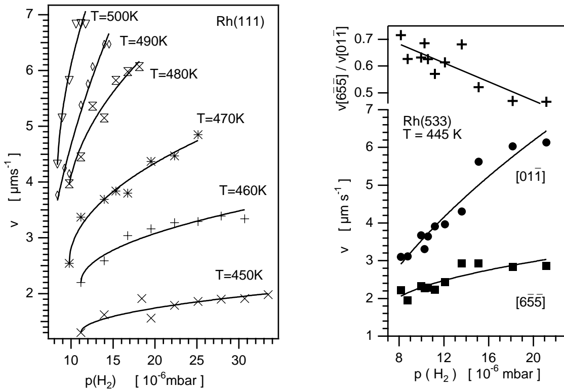
Abbildung 4.8: Geschwindigkeit der chemischen Wellen in der \text{NO} + \text{H}_2 -Reaktion auf Rh(111) und Rh(533). Experimentelle Bedingungen: p(\text{NO}) = 1 \cdot 10^{-6} mbar
