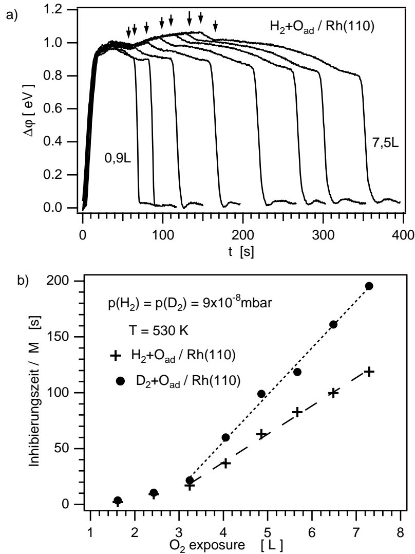
Abbildung 7.10: a) Austrittsarbeitsänderung bei der Dosierung von Rh(110) mit O_2 . Der Pfeil kennzeichnet den Zeitpunkt an dem Sauerstoff abgedreht und p(D_2) = p(H_2) = 9,6 \cdot 10^{-8} \text{ mbar} eingestellt wird. Experimentelle Bedingung: T = 530 \text{ K} , D(O_2) : 1,6 L; 2,4 L; 3,2 L; 4,2 L; 5,0 L; 5,8 L; 6,7 L; 7,6 L b) H/D-Isotopeneffekt in der Inhibierungszeit. Zur Korrektur der unterschiedlichen Auftreffraten wird hier die Inhibierungszeit durch die Wurzel der Masse geteilt.
