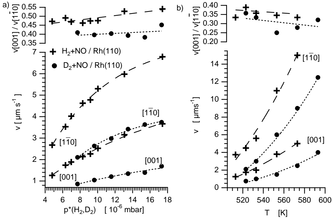
Abbildung 7.7: H/D-Isotopeneffekt in der Puls geschwindigkeit der Reaktion \text{NO} + \text{H}_2/\text{Rh}(110) (a) in Abhängigkeit von p^*(\text{H}_2/\text{D}_2) und (b) in Abhängigkeit von der Temperatur. Experimentelle Bedingungen: p(\text{NO}) = 1,6 \cdot 10^{-6} mbar, a) T = 530 K, b) p^*(\text{H}_2) = p^*(\text{D}_2) = 1 \cdot 10^{-5} mbar
