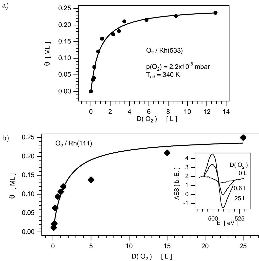
Abbildung 3.6: Zusammenhang zwischen Bedeckung und Sauerstoffdosis. Experimentelle Bedingungen: Rh(533): T_{\text{ad}} = 340 \text{ K} , Rh(111) T_{\text{ad}} = 450 \text{ K}
