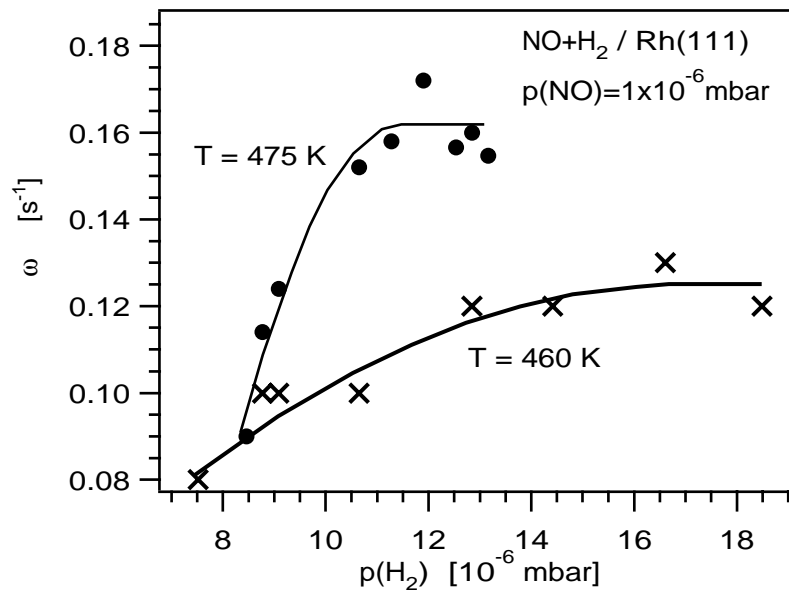
Abbildung 4.13: Abhängigkeit der Spiralfrequenz von p(\text{H}_2) . Experimentelle Bedingungen: p(\text{NO}) = 1 \cdot 10^{-6} mbar
