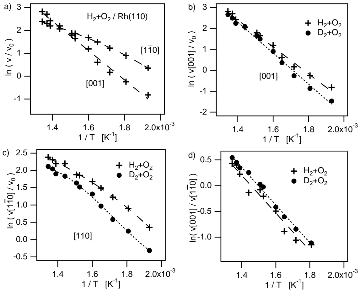
Abbildung 7.9: a) Arrheniusdarstellung der Frontgeschwindigkeit in der Reaktion \text{O}_2 + \text{H}_2 / \text{Rh}(110) (b),(c) H/D-Isotopeneffekte bei der Temperaturabhängigkeit der Frontgeschwindigkeit und d) in der Anisotropie. Experimentelle Bedingungen: p(\text{O}_2) = 2,2 \cdot 10^{-6} mbar, p^*(\text{H}_2) = p^*(\text{D}_2) = 4,3 \cdot 10^{-6} mbar
