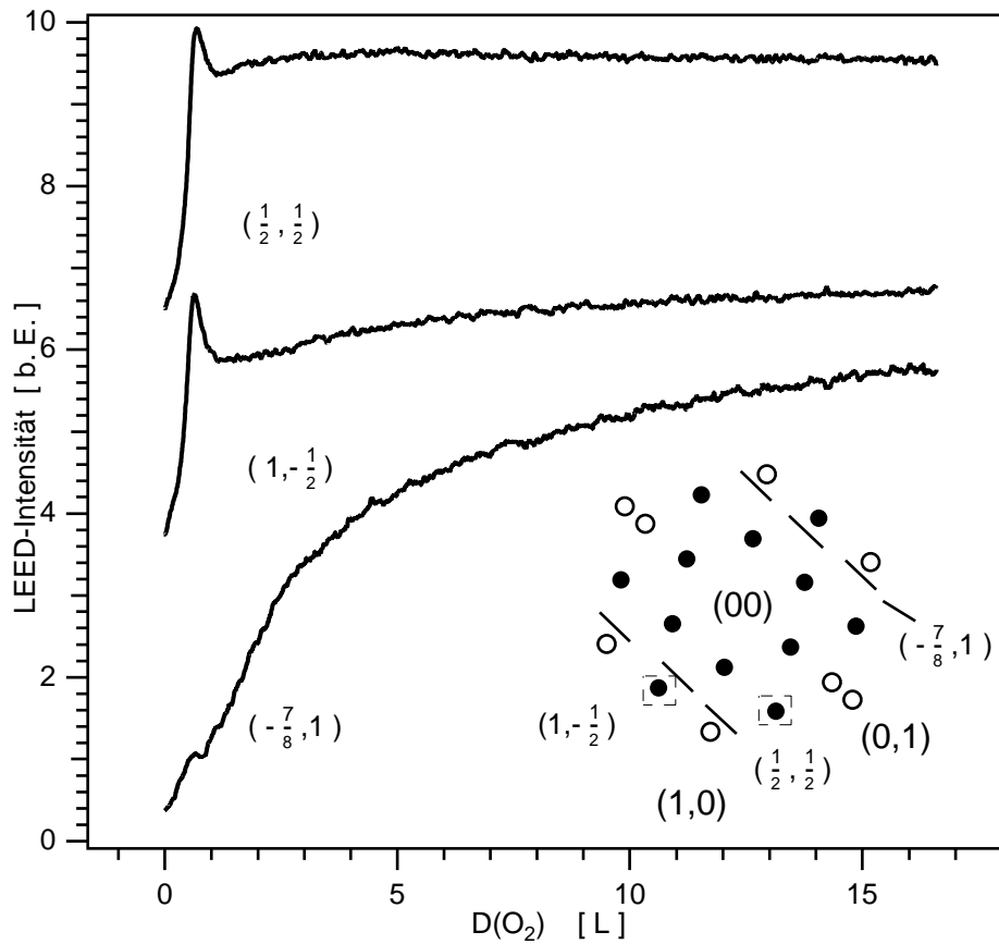
Abbildung 3.5: Entwicklung der LEED-Überstrukturreflexe während der Dosierung von Rh(533) mit Sauerstoff. Reflexe des Grundgitters sind durch Ringe, die der Überstruktur durch schwarze Kreise dargestellt.
