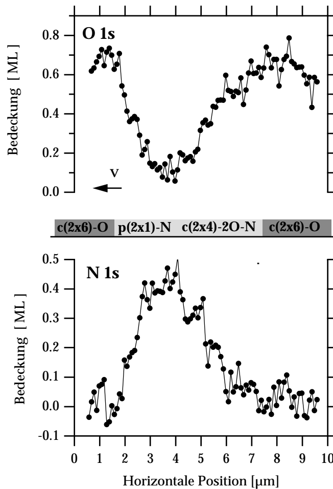
Abbildung 9.4: Absolute Bedeckungen von adsorbiertem Sauerstoff und Stickstoff innerhalb eines Pulses in der Reaktion \text{NO} + \text{H}_2 / \text{Rh}(110) . Die Pulsgeschwindigkeit beträgt v = 0.1 \mu\text{m}/\text{s} . Experimentelle Bedingungen wie in Abbildung 9.2
