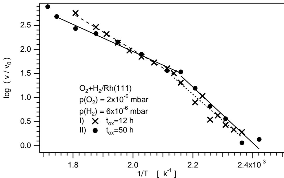
Abbildung 6.9: Temperaturabhängigkeit der Frontgeschwindigkeit der Reaktion O_2+H_2 für zwei verschieden lang oxidierte Oberflächen. Experimentelle Bedingung: I) t_{ox} = 12 h, II) t_{ox} = 50 h, \beta = 8, 1 K/s
