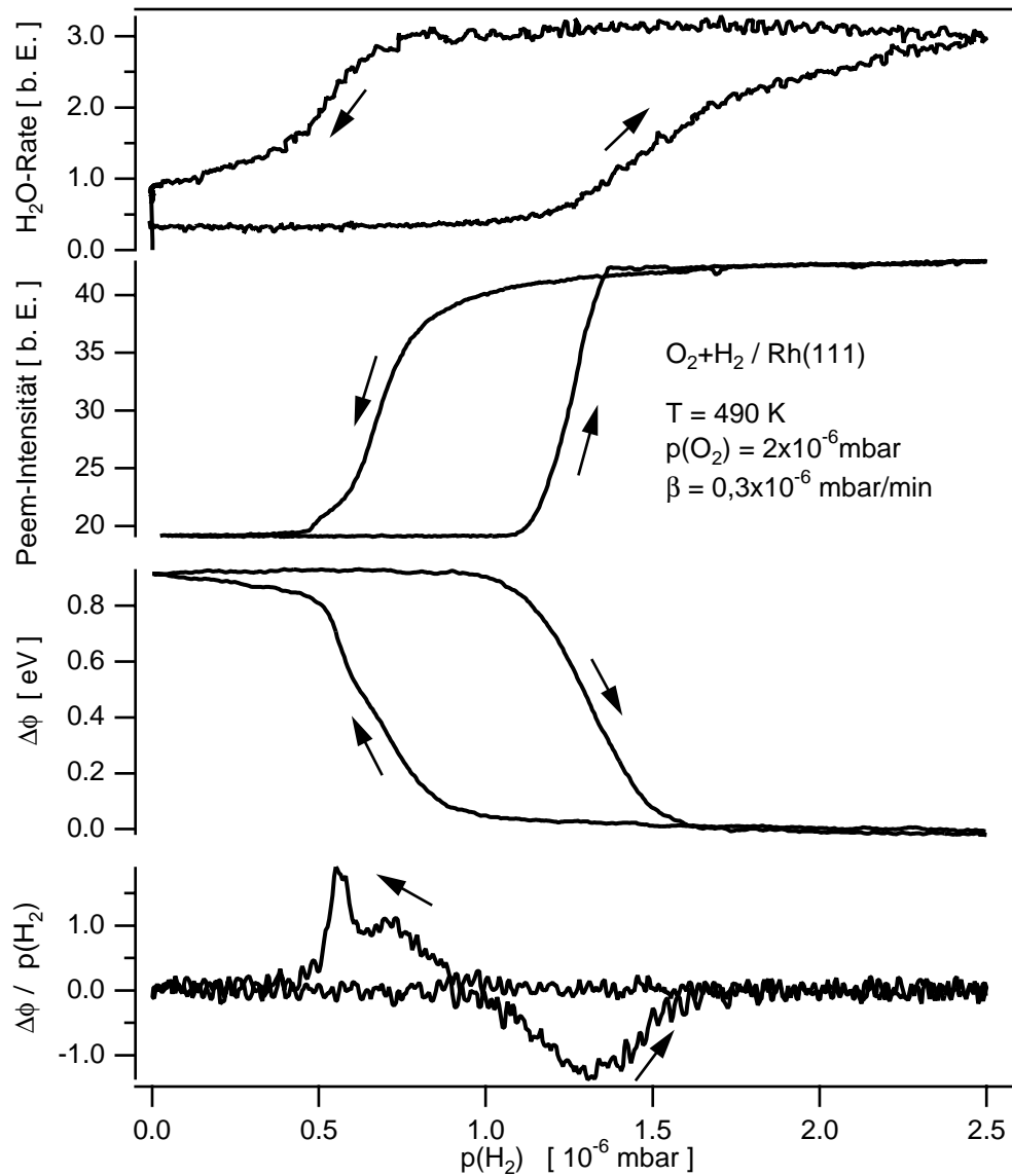
Abbildung 3.10: Dargestellt sind die Hysterese der Ratenproduktion, der PEEM-Intensität und der Austrittsarbeit bei zyklischer Variation von p(\text{H}_2) . Im unteren Teil ist noch die Ableitung der Hysterese der Austrittsarbeit nach p(\text{H}_2) abgebildet.
