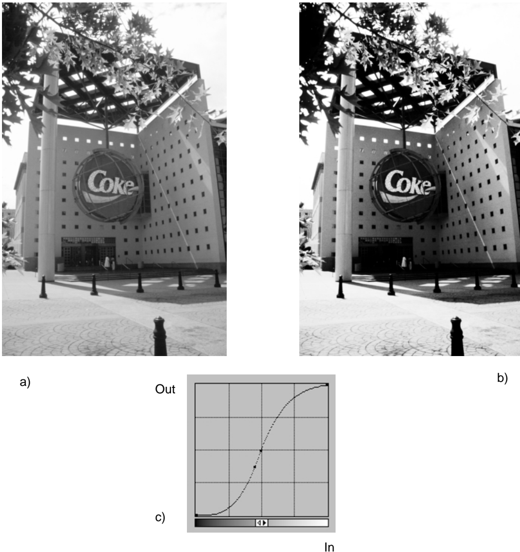
Abb. 4.2: Darstellung der Kontrastanhebung am Beispiel eines Grauwertbildes.
