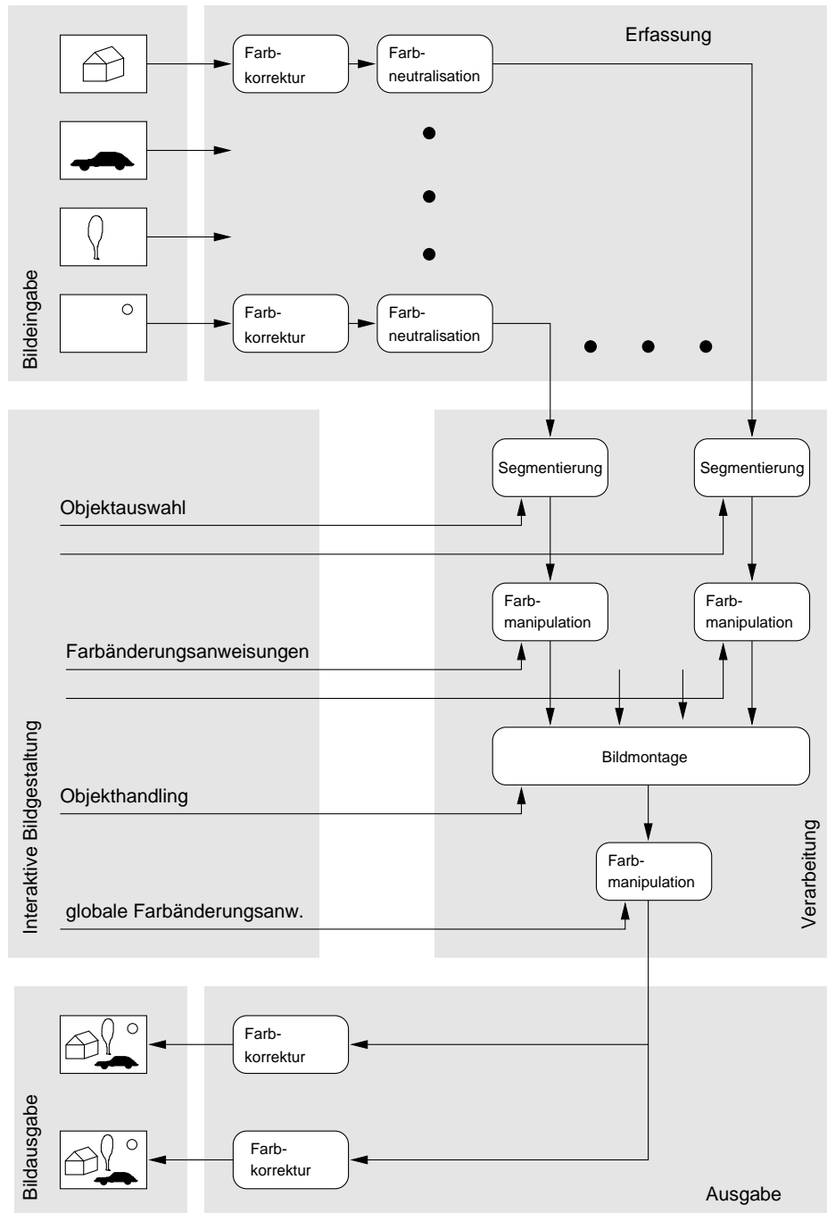
Abb. 3.6: Globale Systemarchitektur und Datenfluß unter Berücksichtigung einer Bildmontage. Die interaktive Farbmanipulation ist Teil des Bearbeitungspfad, während Farbkorrektur und Farbneutralisation automatisch ablaufen und daher der Bilderfassung zugeordnet werden können.
