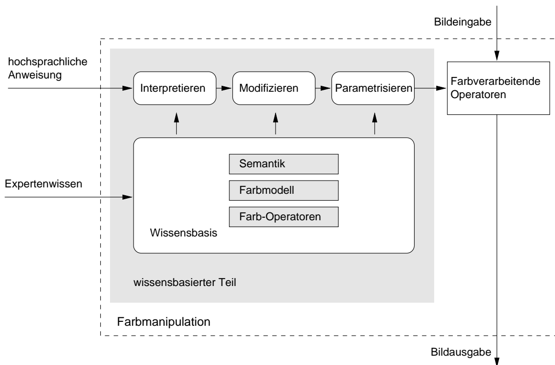
Abb. 4.5: Systemarchitektur der Farbmanipulation Die farbverarbeitenden Operatoren sind Teil des Bearbeitungspfades.
