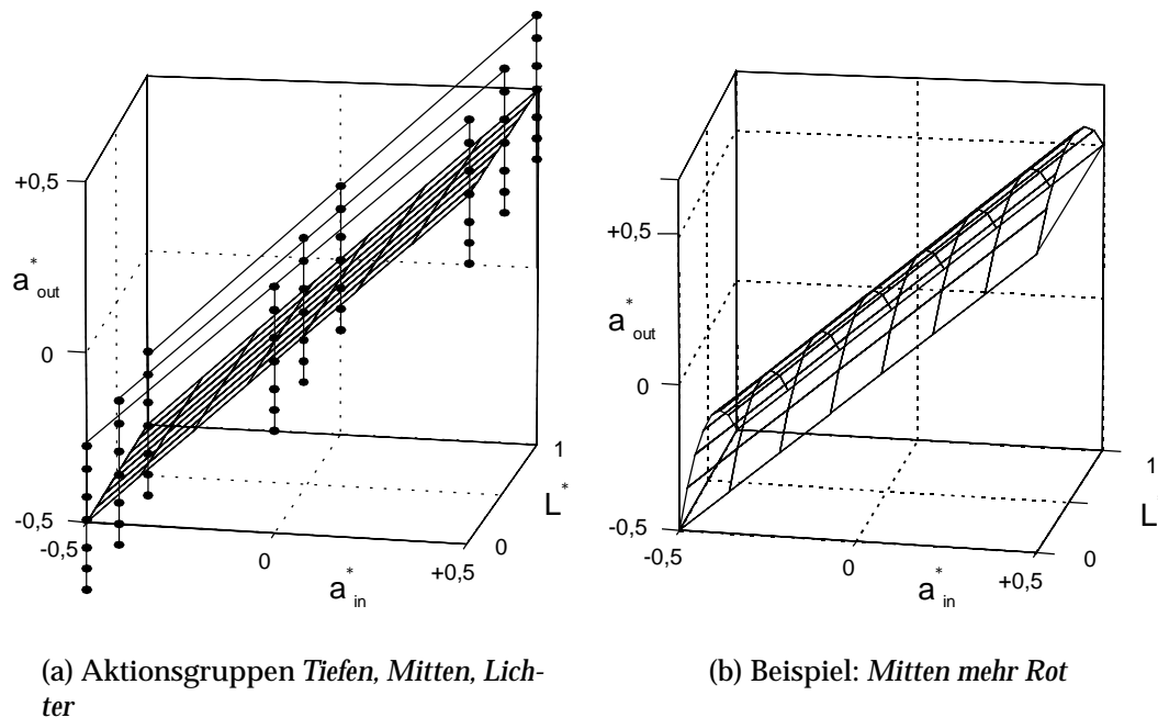
Abb. 4.11: Tonwertabhängige Farbmanipulation
