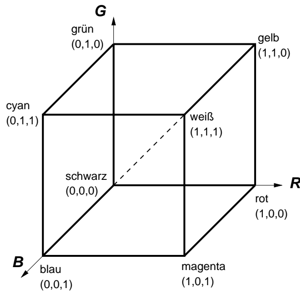
Abb. 2.5: Das RGB-Farbmodell.
