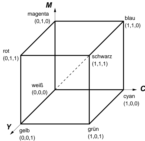
Abb. 2.6: Das CMY-Farbmodell.
