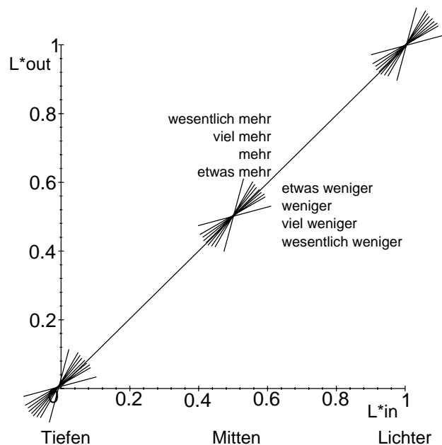
Abb. 4.9: Die tonwertabhängige Kontrastmanipulation erfolgt durch Vorgabe der gewünschten Kontraständerung für jeden Aktionsbereich (Tiefen, Mitten, Lichter). Entsprechend kann die Steigung an diesen Punkten der Funktion vorgegeben werden. Die Steigung 1 läßt den Kontrast unverändert. Höhere Werte verstärken, niedrigere Werte flachen den Kontrast ab. Sinngemäß zu Abb. 4.7 werden auch hier die Begriffe aus Tab. 4.2 verwendet.
