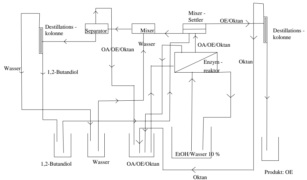
Abbildung 6-1: Vorschlag zur Reaktionsführung, um mit einer extraktiven, enzymatischen Veresterung kontinuierlich Carbonsäureethylester zu gewinnen.
