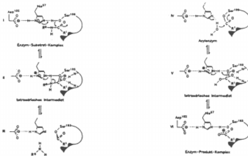
Abbildung 2-6: Mechanismus der Proteinspaltung durch Trypsin [48].
