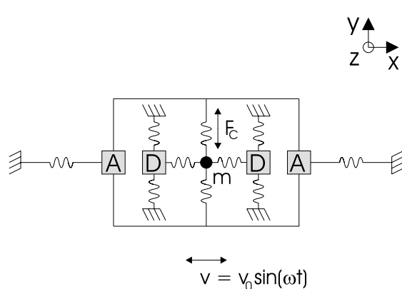
Abbildung 3.2: Schematischer Aufbau eines Einmassenschwingers mit eingezeichneten Aktoren A und Detektoren D , die von der Schwingung der seismischen Masse in y -Richtung bzw. in x -Richtung entkoppelt sind.
