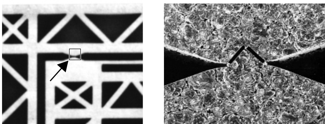
Abbildung 5.4: Anschlag der seismischen Masse. Zur Orientierung ist links ein Detailausschnitt aus Abb. 5.2 dargestellt. Der eingerahmte Bereich ist rechts für einen Sensor mit einer Detektorspaltweite von 2 \mu\text{m} vergrößert wiedergegeben. Die seismische Masse und der Sensorrahmen sind miteinander verbunden.
