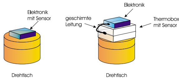
Abbildung 6.9: Bei der Bestimmung der Temperaturabhängigkeit der Steilheit und des Offsets enthält die Elektronik nicht mehr das Sensorelement (links), sondern das über eine geschirmte Leitung mit der Elektronik verbundene Sensorelement wird in einer Thermobox passiv temperiert.
