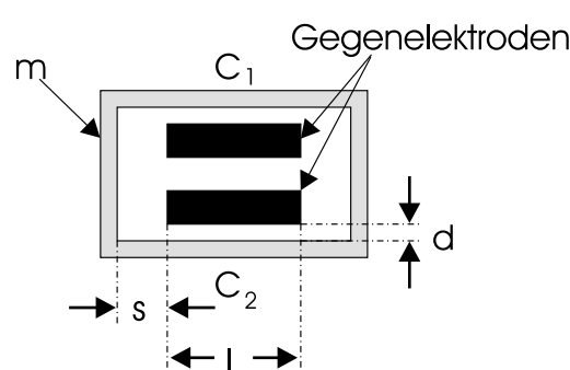
Abbildung 3.5: Vergrößerte Darstellung der seismischen Masse m .
