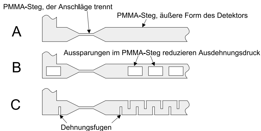
Abbildung 7.1: PMMA-Form des Detektoranschlages. A: Aktuelles Design. B,C: Varianten zur Reduzierung des thermisch induzierten Drucks auf den dünnen PMMA-Steg, der die Anschlüsse voneinander trennt.
