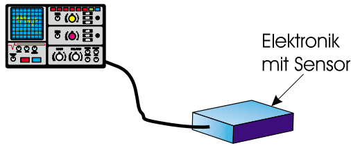
Abbildung 6.5: Meßaufbau zur Bestimmung des Rauschsignals \Omega_n über das Rauschspektrum der Sensorelektronik.
