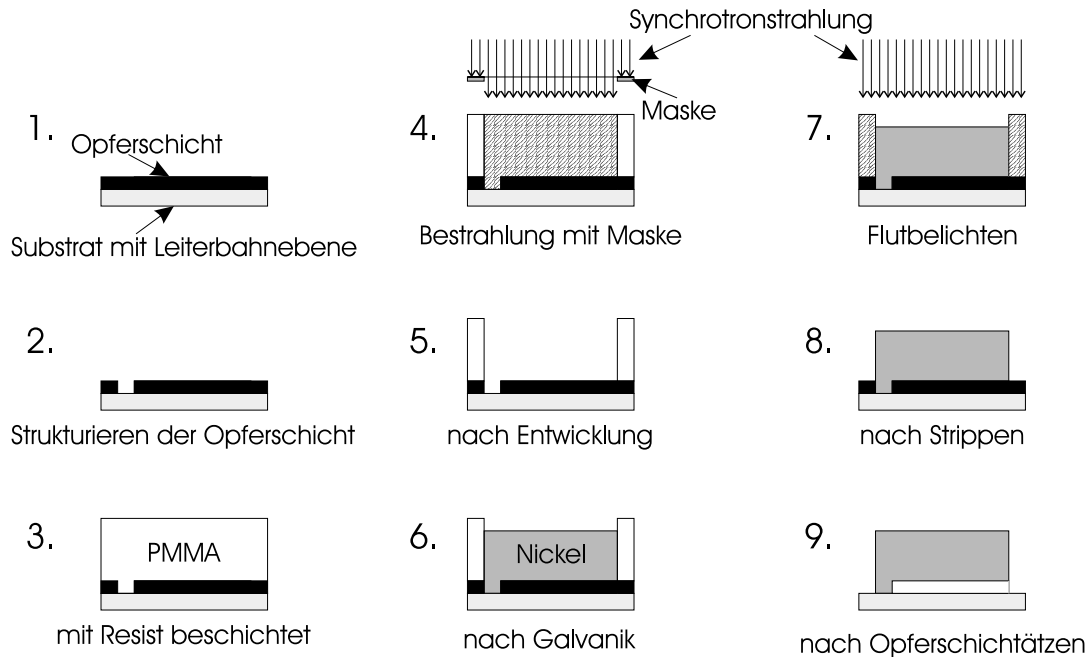
Abbildung 2.4: Prozessabfolge des LIGA-Verfahrens.
