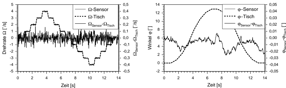
Abbildung 6.14: Links: Drehrate des Sensors und des Drehtisches sowie deren Differenz. Rechts: Aus der Drehrate berechneter Winkel des Sensors und des Drehtisches und deren Abweichung.
