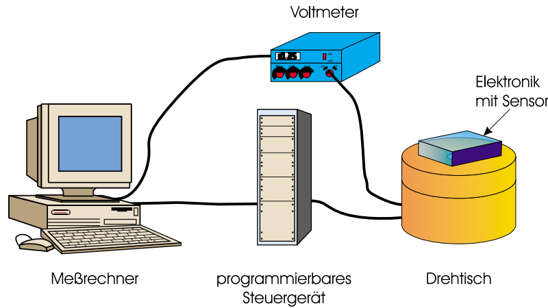
Abbildung 6.1: Meßaufbau für Linearitäts-, Drift- und Winkelmessungen. Über einen Meßrechner wird das Steuergerät des Drehtischs programmiert. Die Sensorspannungssignale werden von einem Voltmeter bestimmt und an den Meßrechner weitergegeben.
