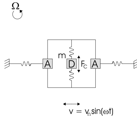
Abbildung 3.3: Aufbau des Sensors mit einem in die seismische Masse m integrierten Detektor D .
