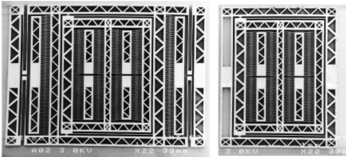
Abbildung 5.2: REM-Bilder des LIGA-Gyrometers und des an das Gyrometer angepassten LIGA-Beschleunigungssensors.
