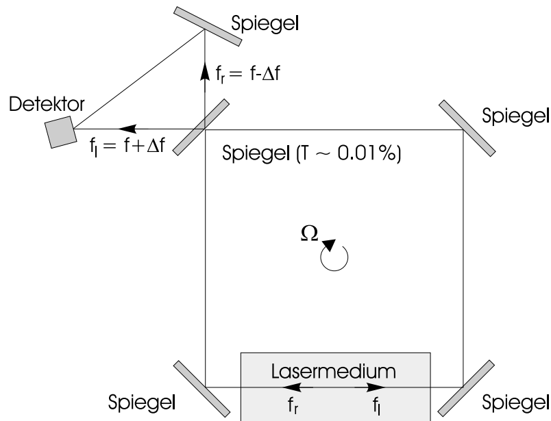
Abbildung 1.5: Aufbau eines einfachen Ringlaser-Gyrometers. Durch stimulierte Emission werden in dem lasernden Medium zwei Laserstrahlen erzeugt, die in zueinander entgegengesetzter Richtung den aus vier Spiegeln bestehenden Resonator durchlaufen. Ein kleiner Teil der Laserstrahlen tritt aus dem Resonator aus und wird auf den Detektor gelenkt, wo die beiden Laserstrahlen interferieren.
