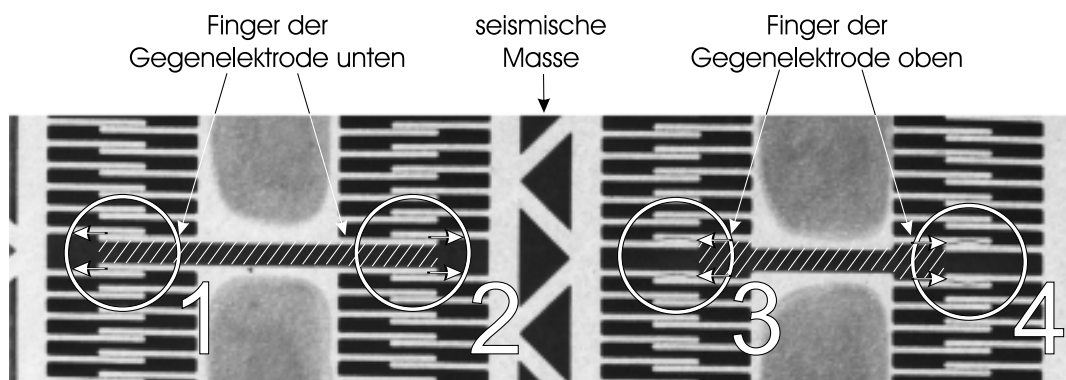
Abbildung 5.3: Mittlerer Teil des Detektors mit einer Detektorspaltweite von 3 \mu\text{m} . Die inneren Fingerelektroden der Ringe 3 und 4 sind verbogen. Die Fingerelektroden der Ringe 1 und 2 weisen keine derartigen Verbiegungen auf. Ursache hierfür ist der weiß gestrichelte Bereich.
