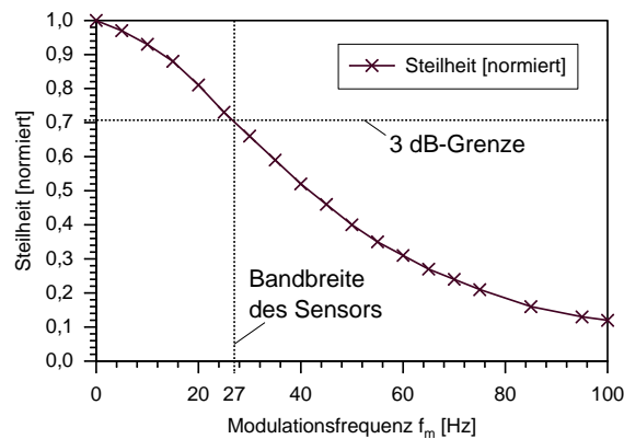
Abbildung 6.4: Abhängigkeit der Steilheit von der Modulationsfrequenz f_m .
