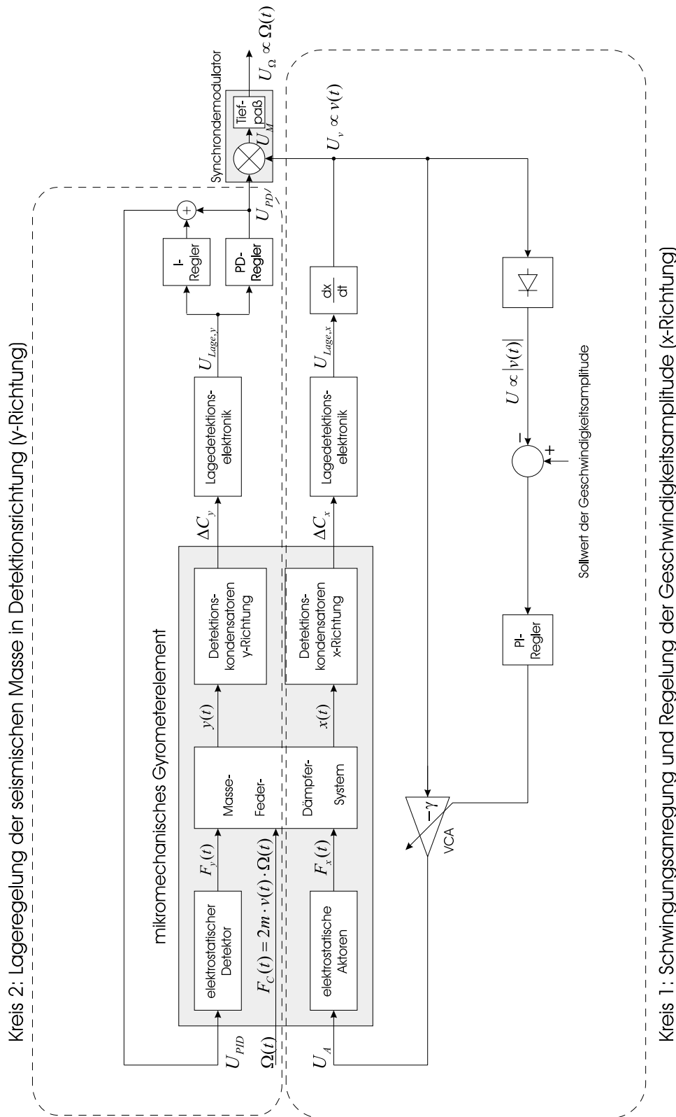
Abbildung 5.13: Blockschaltbild der Auswerteelektronik.
