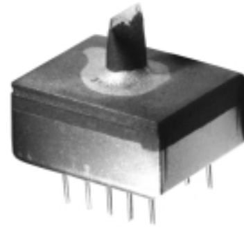
Abbildung 5.11: Lasergeschweißtes, ausgepumptes und abgepitchtes Gehäuse.
