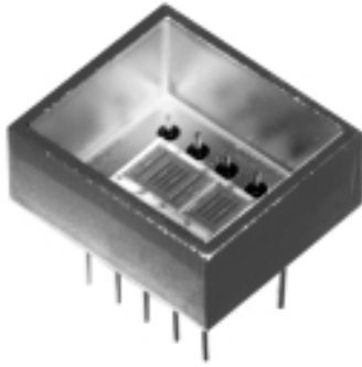
Abbildung 5.9: Eingeklebtes und gebundenes Sensorelement.
