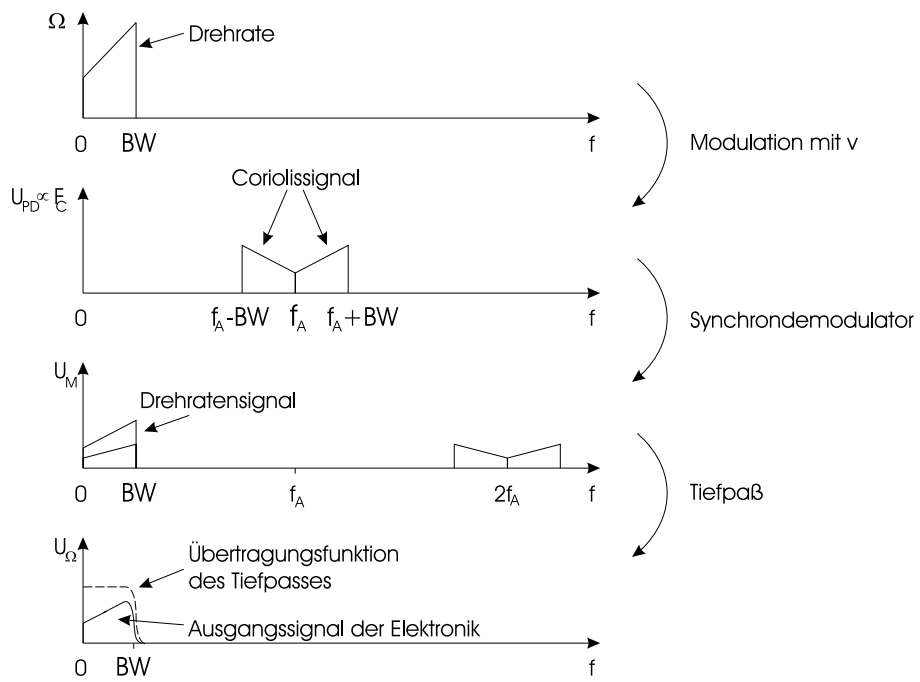
Abbildung 5.14: Frequenzspektren der einzelnen Auswertungsstufen.
