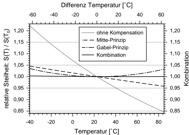
Abbildung 3.10: Die Graphik zeigt den Verlauf von \frac{S(T)}{S(T_0)} über der Temperatur T für die verschiedenen Anordnungen der Gegenelektroden. Die Spaltbreite beträgt 2 \mu\text{m} .
