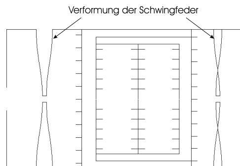
Abbildung 4.3: Darstellung des zweiten dem Anregungs-Oszillator entsprechenden Eigenmode.
