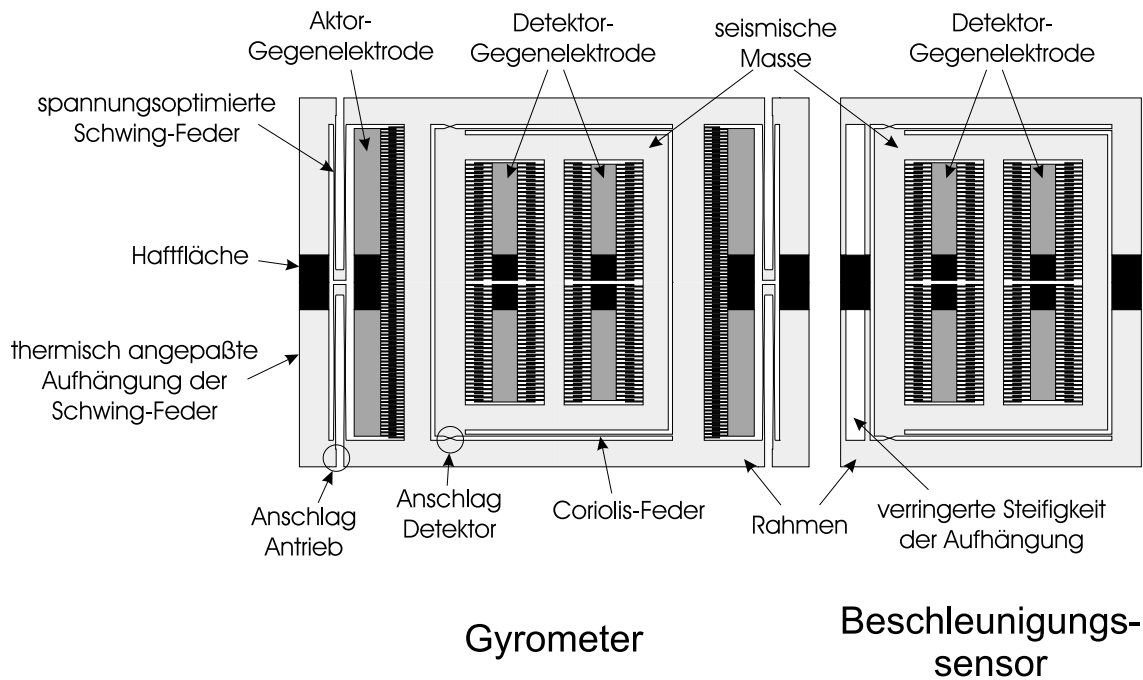
Abbildung 3.22: Mit Hilfe des erstellten Programms erzeugte maßstabsgetreue Darstellung des berechneten Sensors mit einer Kondensatorspaltweite von 4 \mu\text{m} .
