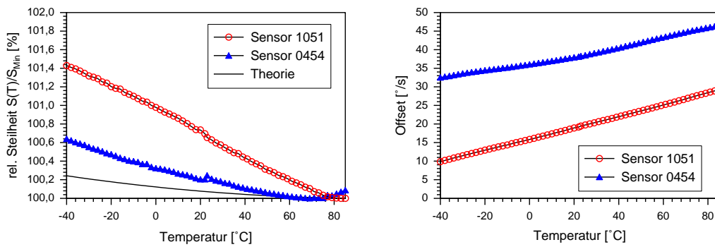
Abbildung 6.10: Temperaturabhängigkeit der Steilheit und des Offsets zweier Sensoren im Vergleich mit der theoretischen Abhängigkeit der Steilheit von der Temperatur.
