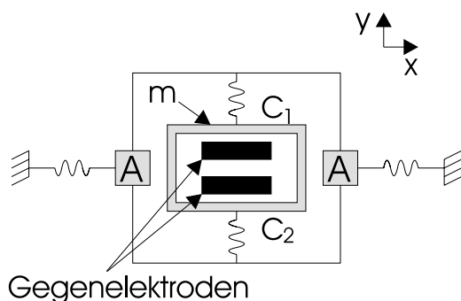
Abbildung 3.4: Aufbau des Gyrometers mit einem in der seismischen Masse m integrierten Detektor.
