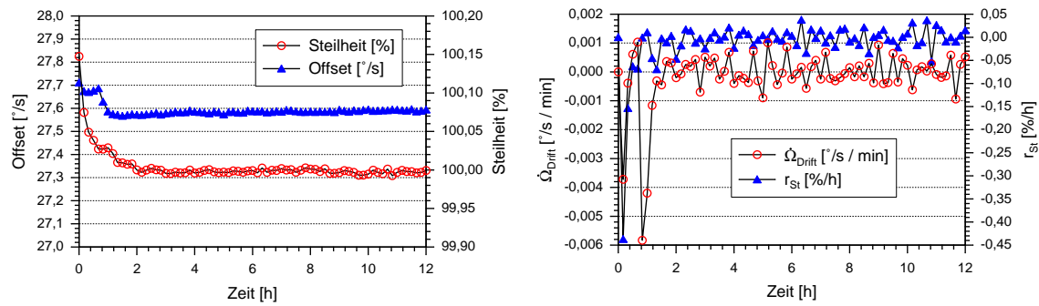
Abbildung 6.12: Links: Drift des Offsets und der Steilheit des Sensors 1051 über einen Zeitraum von zwölf Stunden bei konstanter Außentemperatur (Langzeitdrift). Rechts: Zugehörige differenzielle Drift des Offsets \dot{\Omega}_{Drift} und der Steilheit r_{St} (Kurzzeitdrift).
